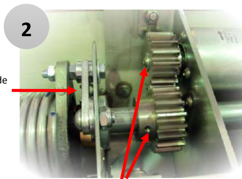
Ressort de rappel Fixations des pignons « moteur » (1 vis axiale) et « arbre » (2 vis radiales à 120°)
